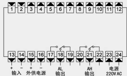
96×48尺寸的仪表:
